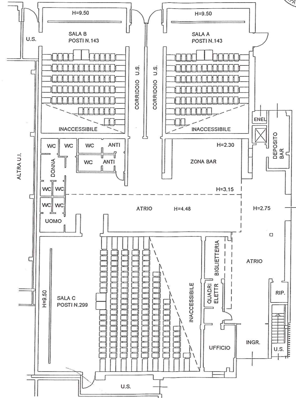
PIANTA PIANTERRENO
