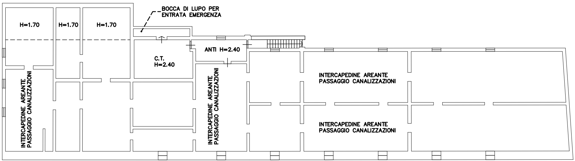
PRIMO INTERRATO H=2.50
