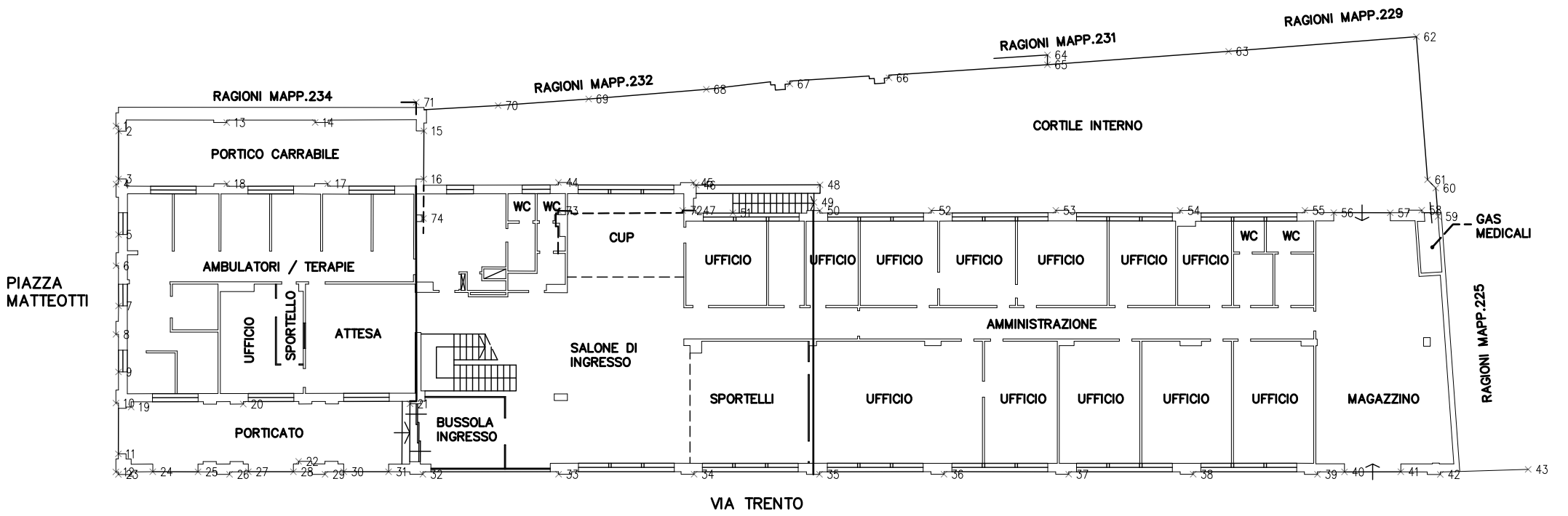
PIANTERRENO H=3.05
