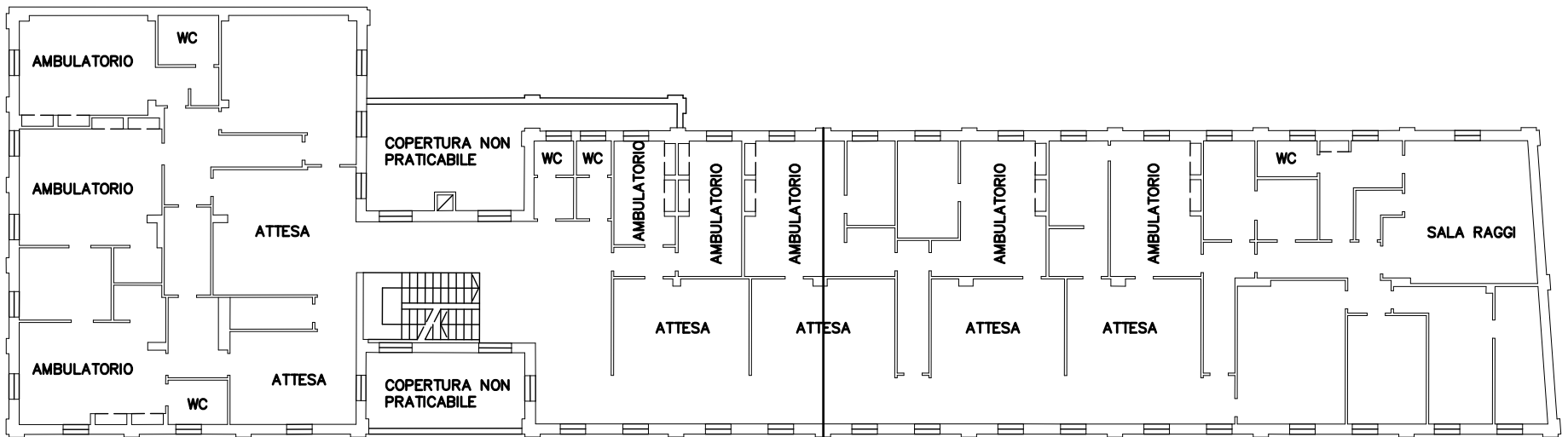
PRIMO PIANO H=3.05
