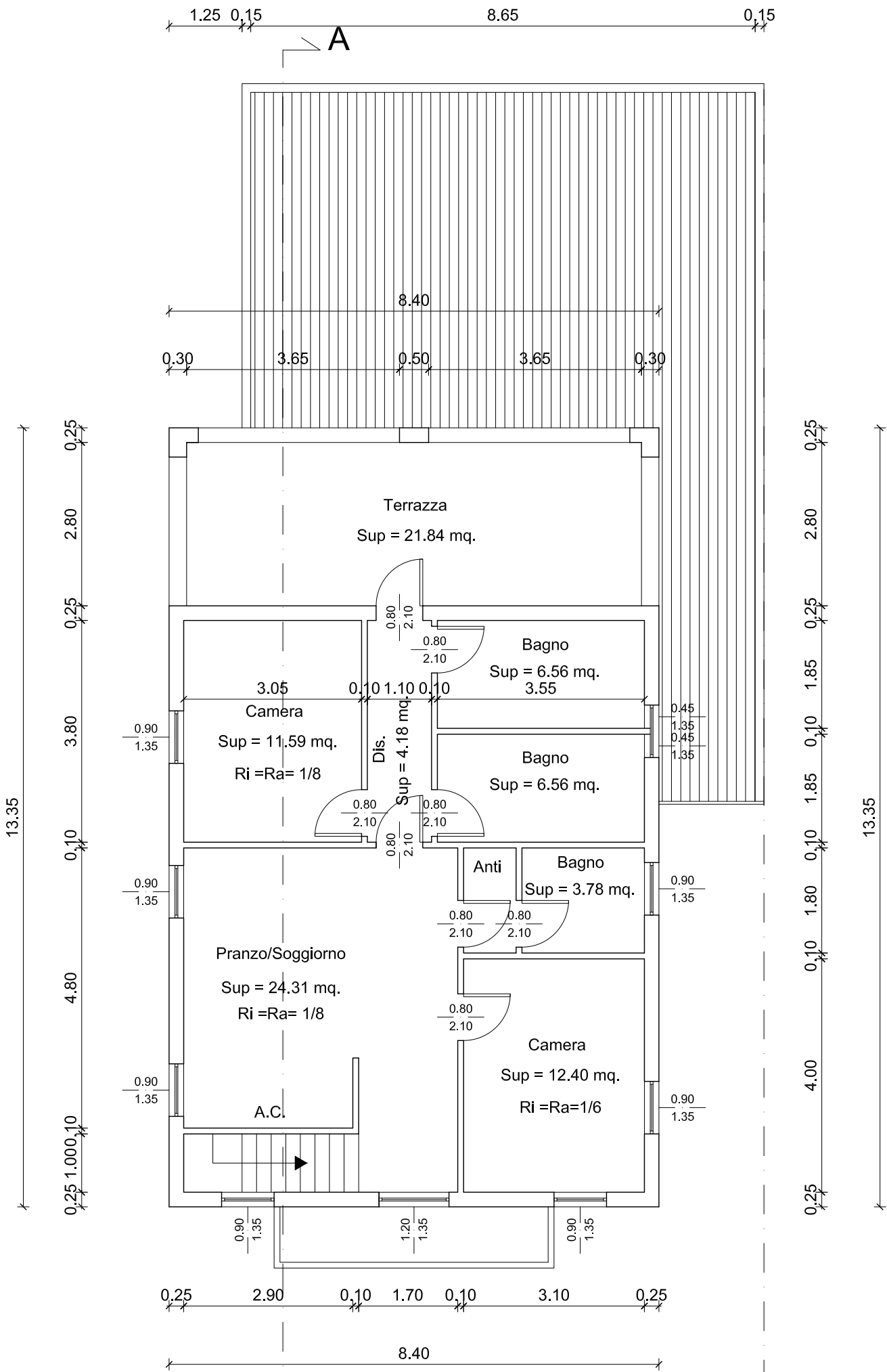
PIANO PRIMO
